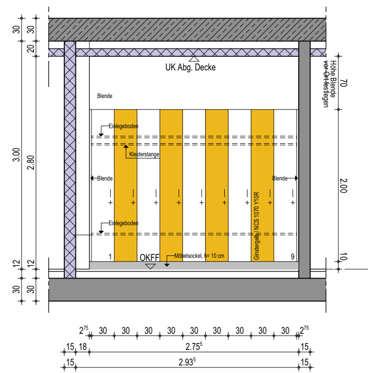
Wandansicht A
