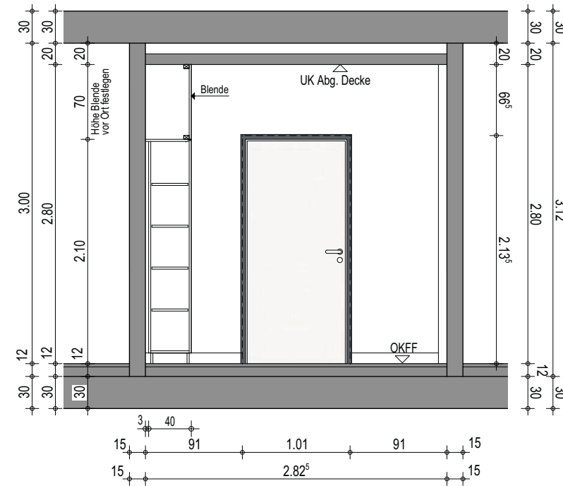
Wandansicht B
