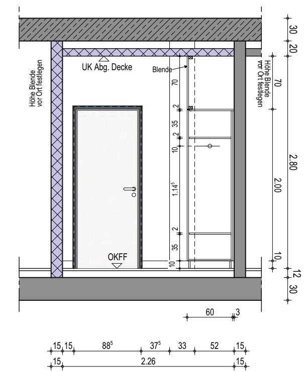
Wandansicht B
