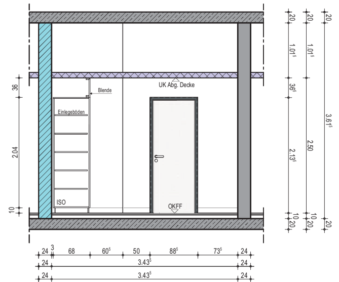
Wandansicht D
