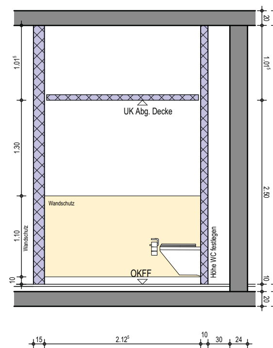
Wandansicht D
