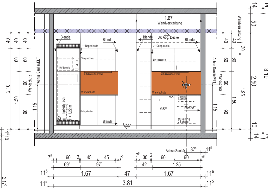
Wandansicht A
