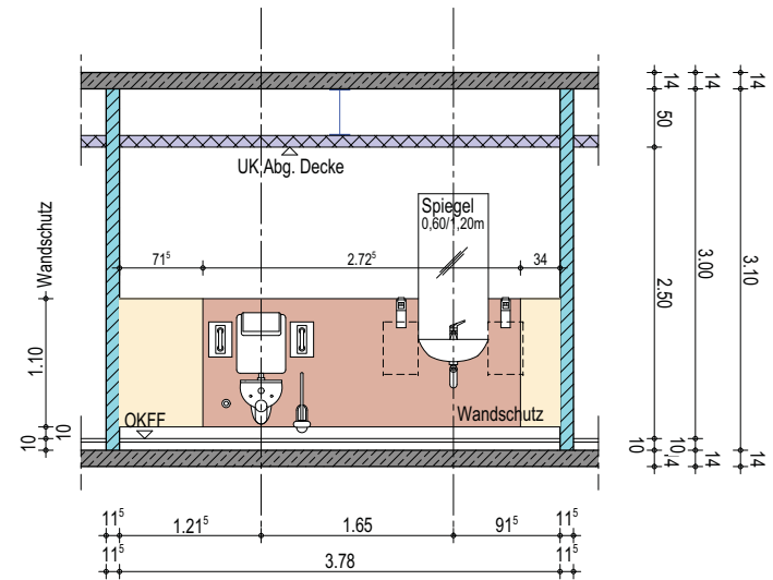
Wandansicht C
