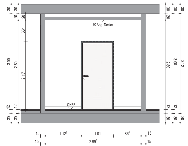
Wandansicht B
