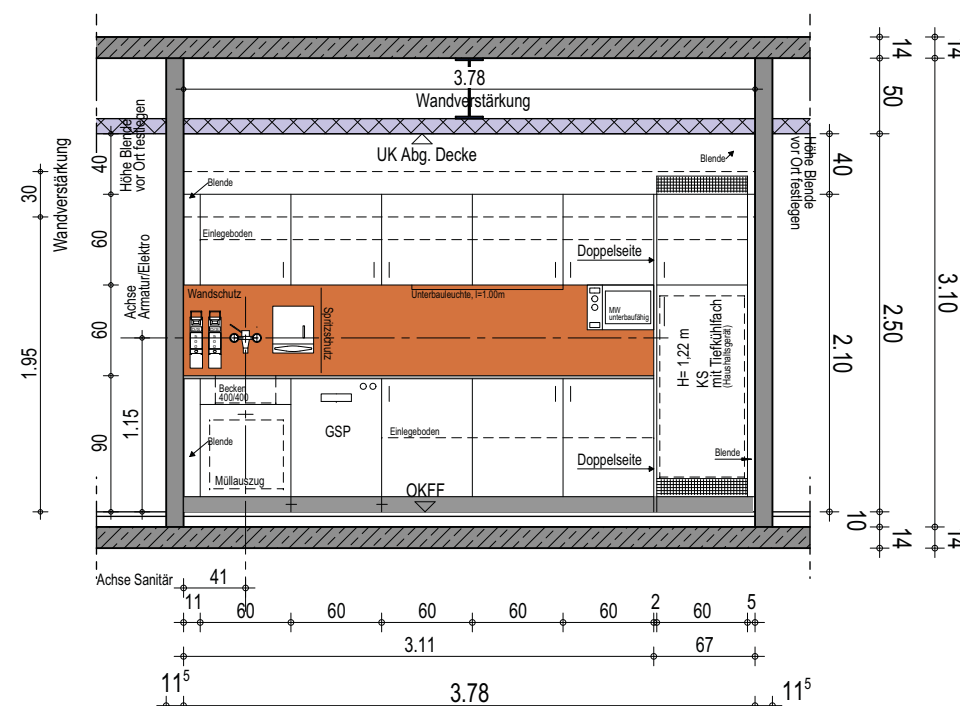
Wandansicht A
