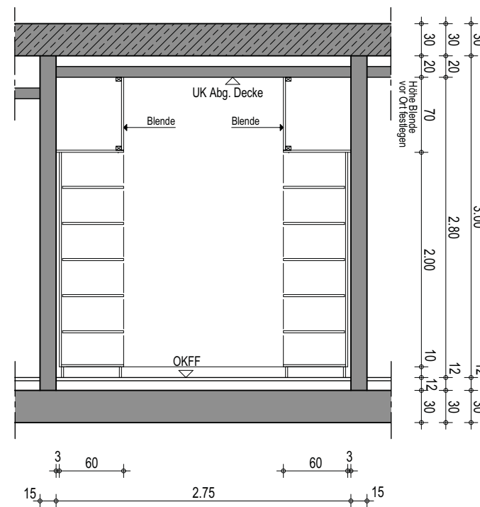
Wandansicht B
