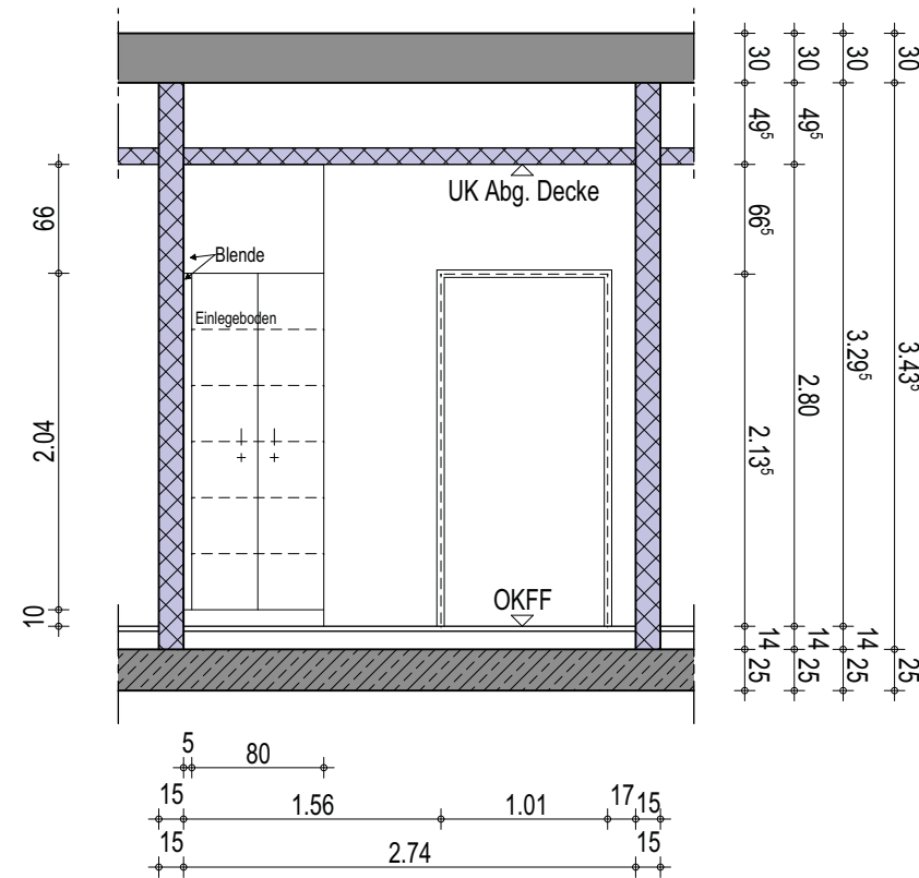
Wandansicht B
