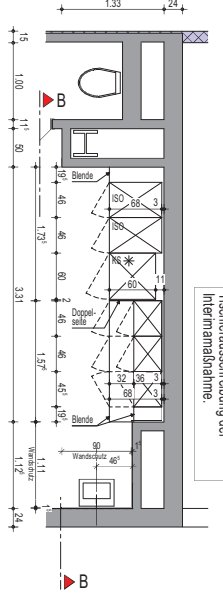
Grundriss Endoskopie
