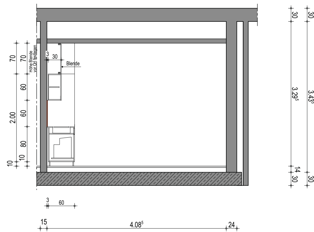
Wandansicht B
