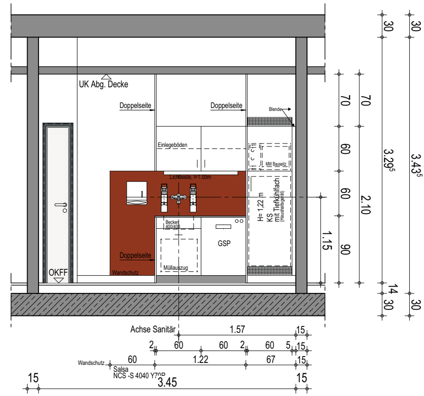
Wandansicht A
