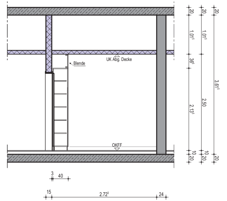
Wandansicht B
