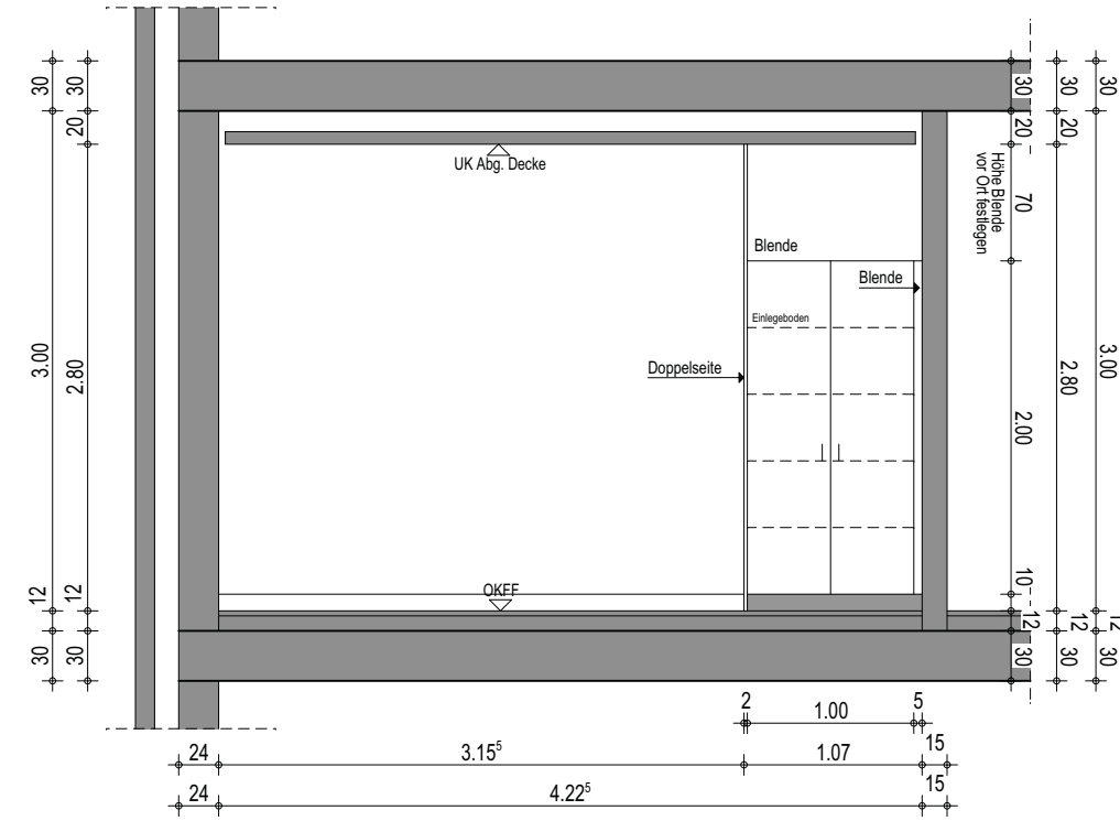
Wandansicht A
