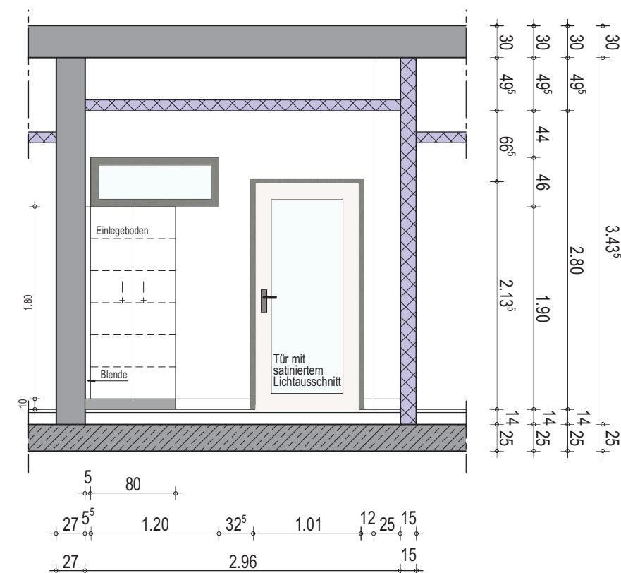
Wandansicht B
