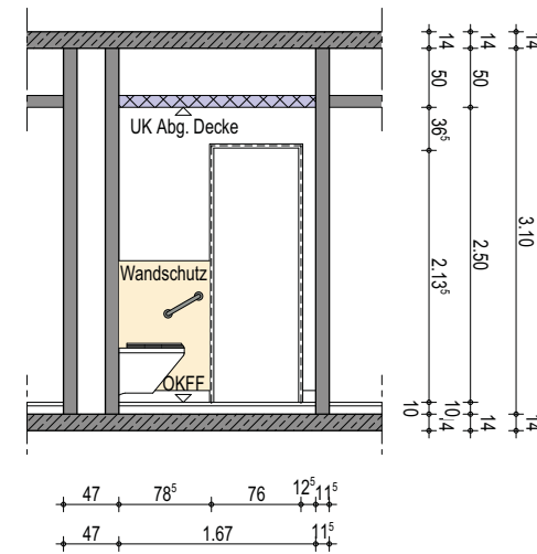
Wandansicht C
