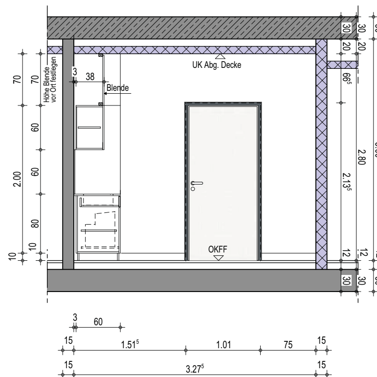
Wandansicht B
