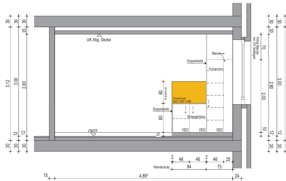
Wandansicht C
