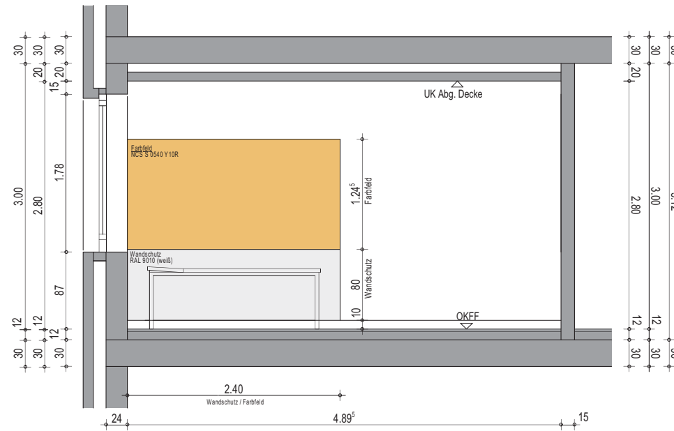
Wandansicht A
