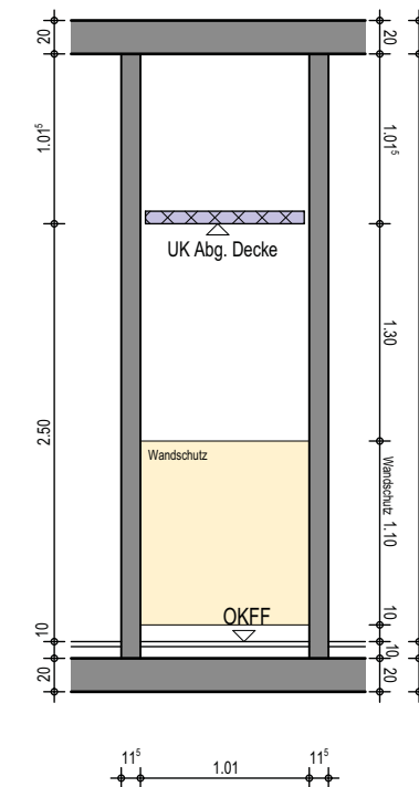
Wandansicht D
