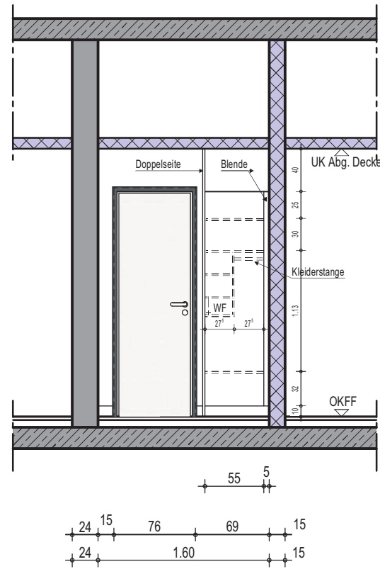
Wandansicht A
