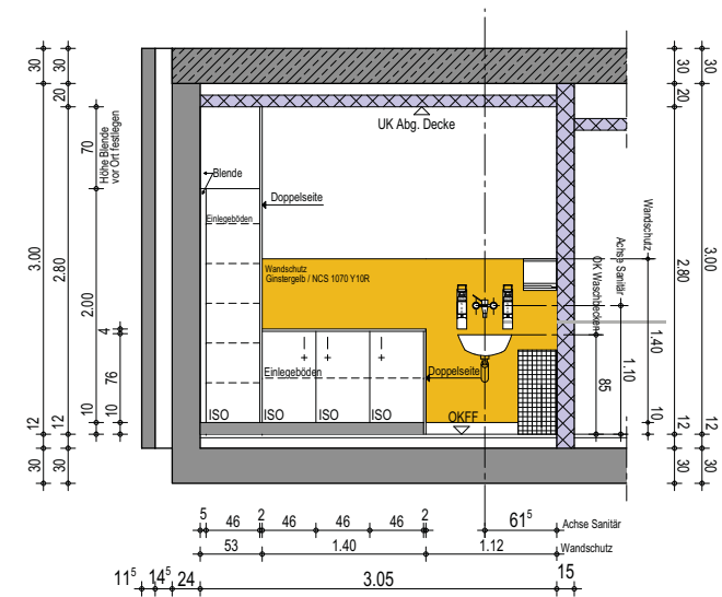
Wandansicht D
