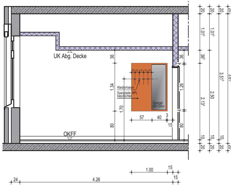
Wandansicht C
