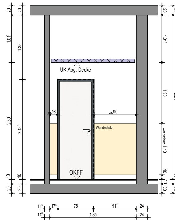
Wandansicht C
