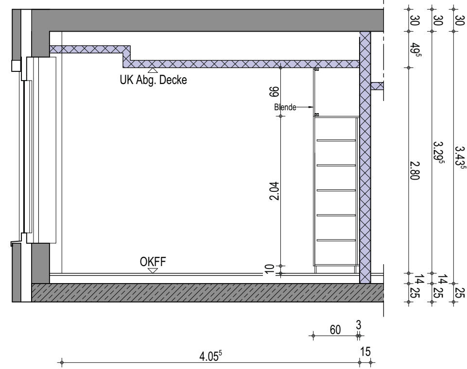
Wandansicht A
