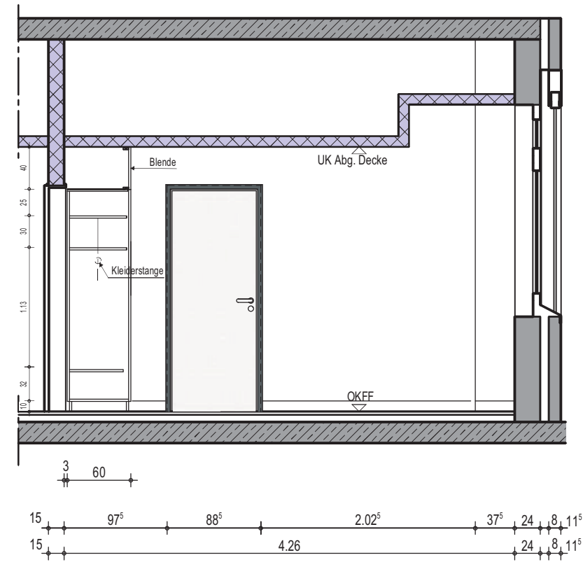
Wandansicht B
