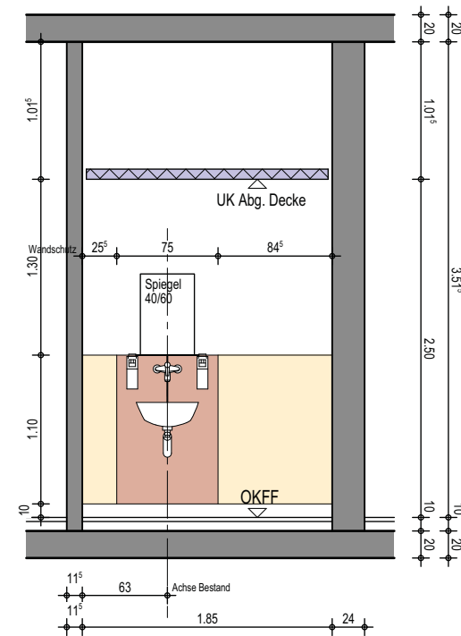
Wandansicht A
