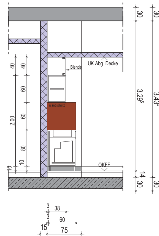
Wandansicht B
