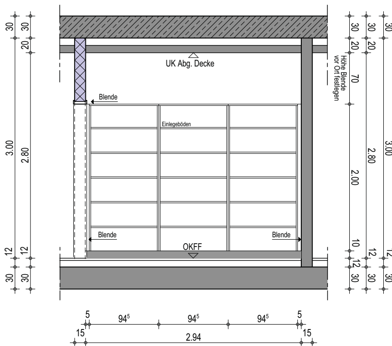
Wandansicht A
