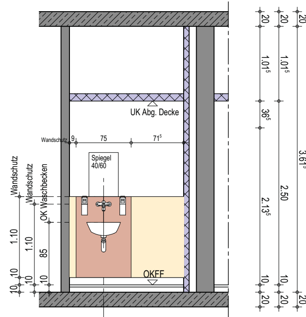
Wandansicht A
