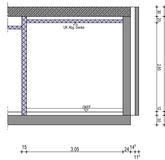
Wandansicht B
