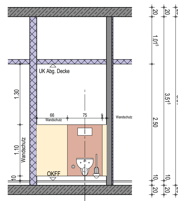
Wandansicht B
