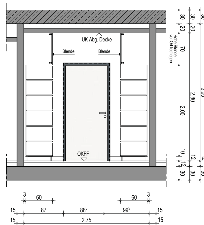
Wandansicht B
