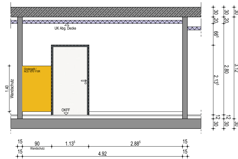
Wandansicht A
