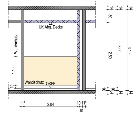
Wandansicht B
