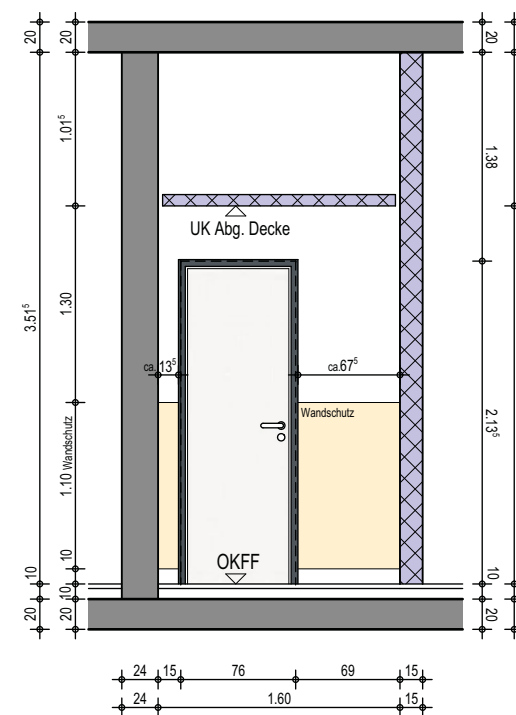
Wandansicht C
