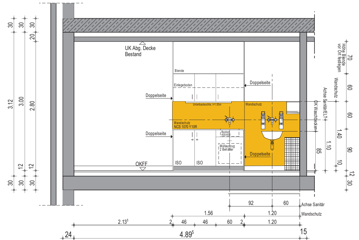
Wandansicht A
