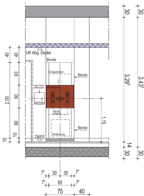
Wandansicht A
