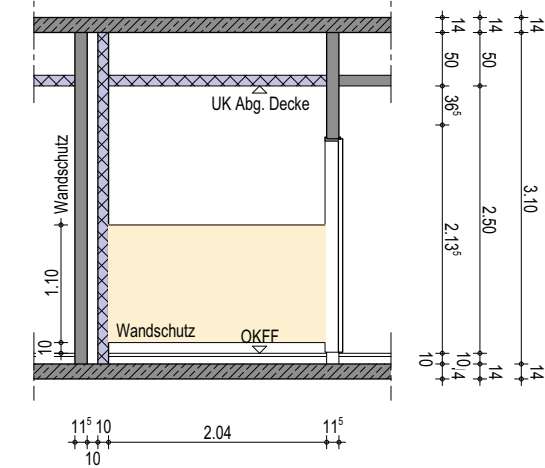
Wandansicht D
