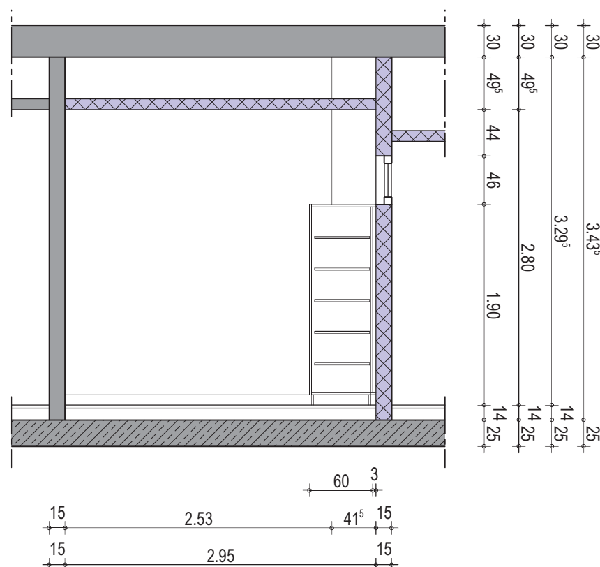
Wandansicht A
