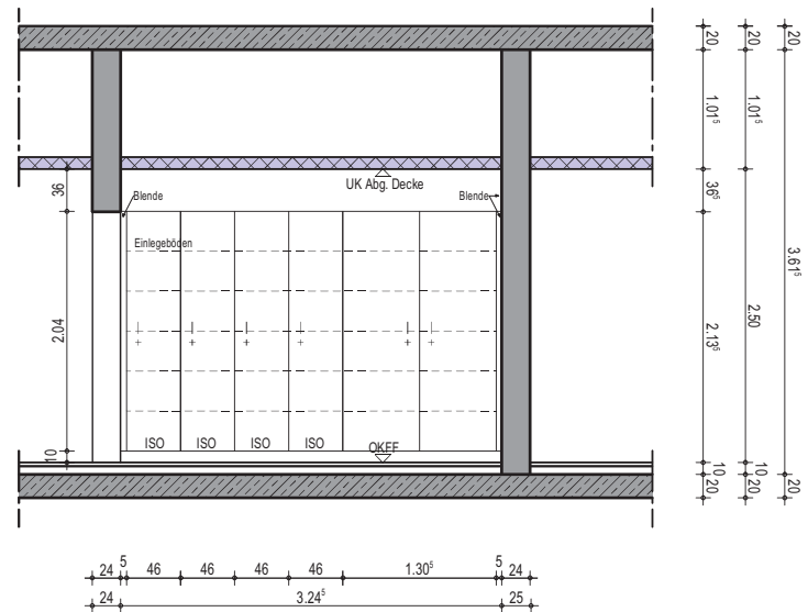
Wandansicht C
