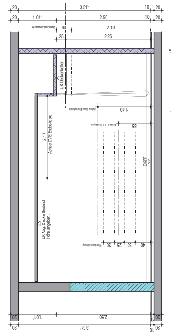
Grundriss Endoskopie
