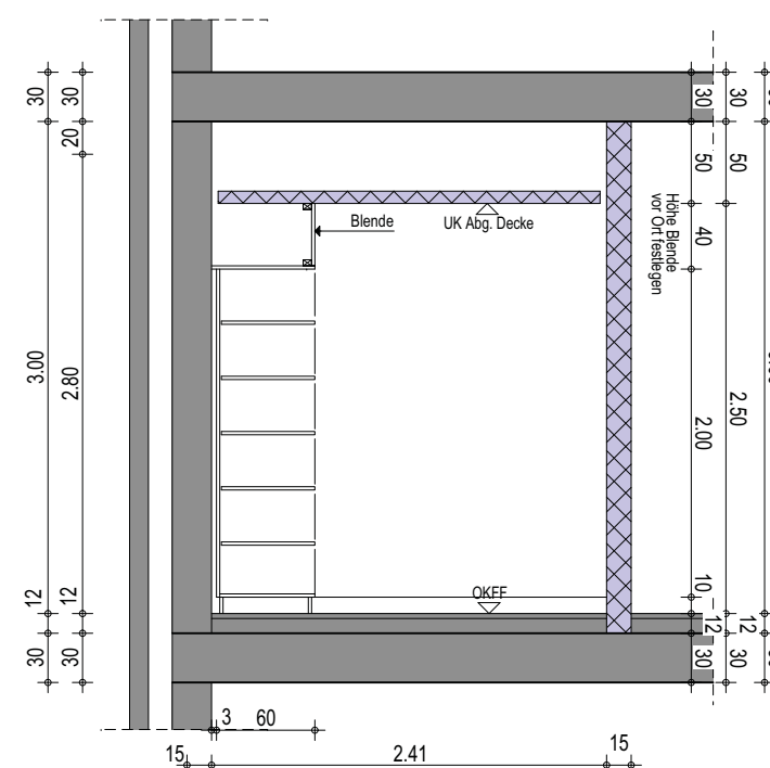
Wandansicht B
