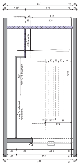
Grundriss Endoskopie
