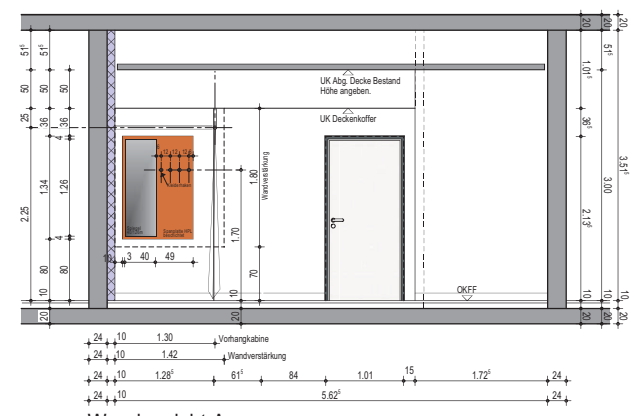
Wandansicht A
