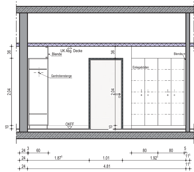
Wandansicht A
