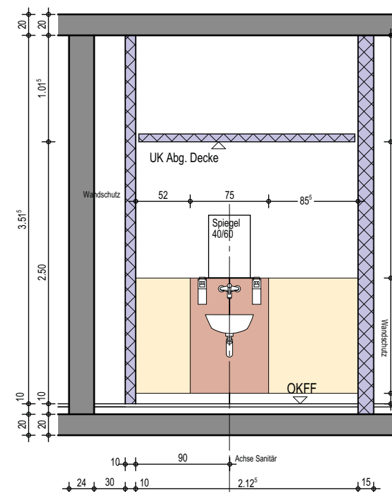
Wandansicht B
