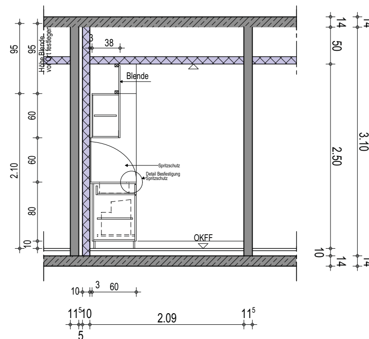
Wandansicht B
