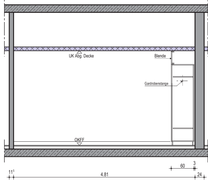
Wandansicht C
