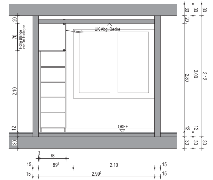
Wandansicht D
