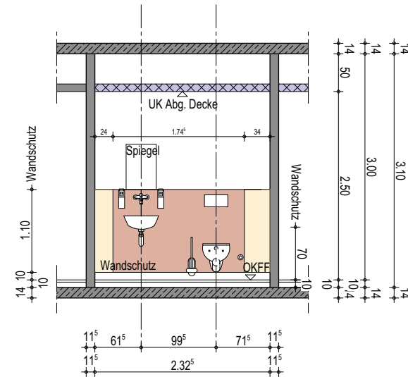
Wandansicht B
