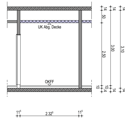
Wandansicht D
