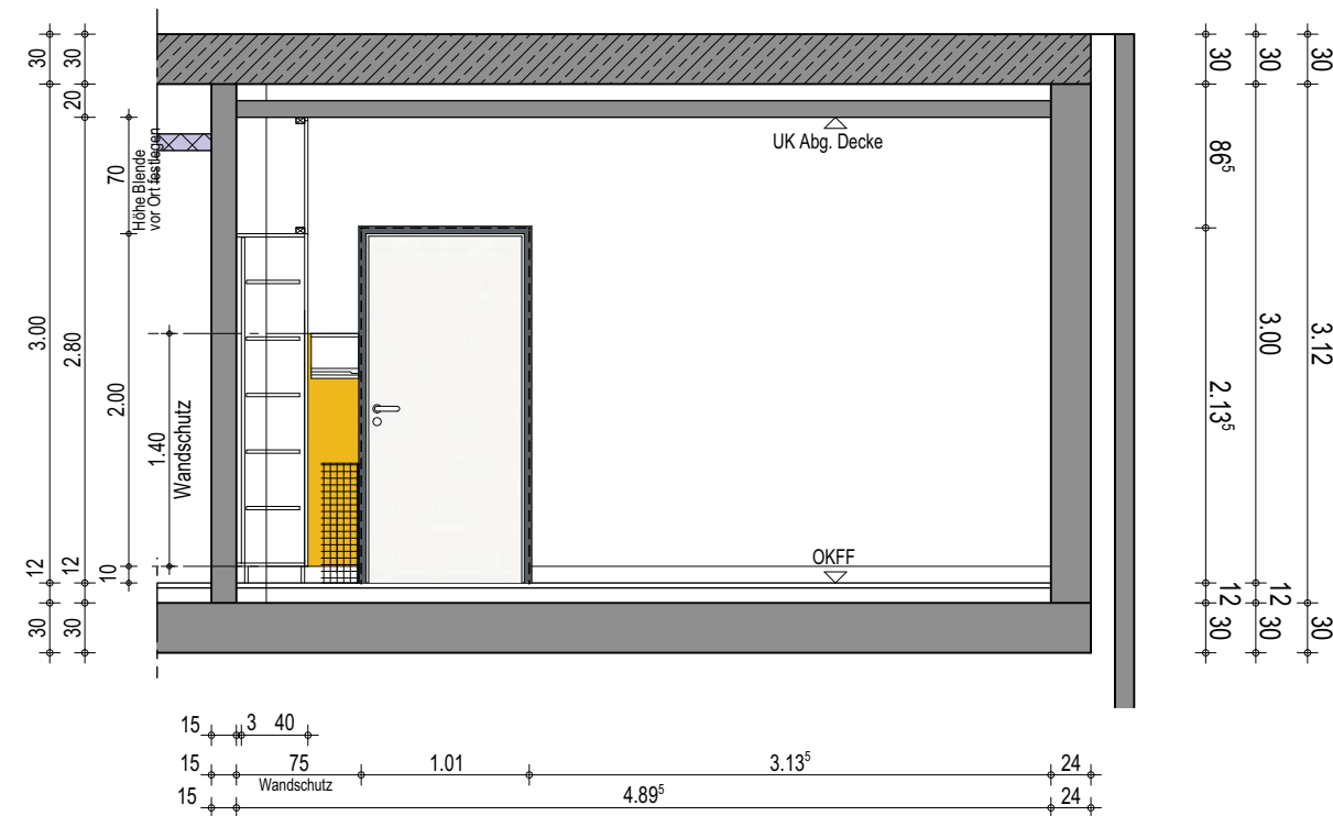
Wandansicht B
