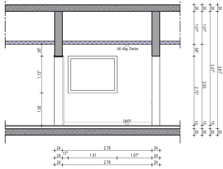
Wandansicht A
