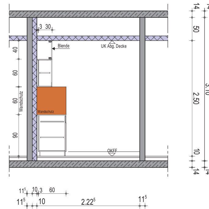
Wandansicht B
