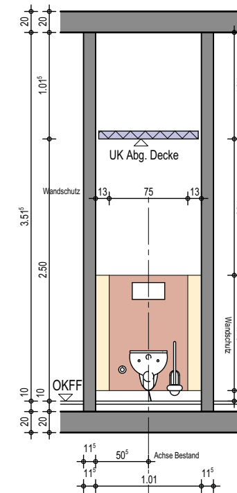
Wandansicht B
