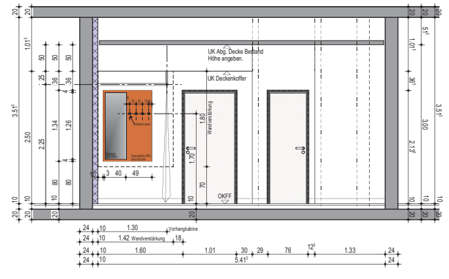
Wandansicht A
