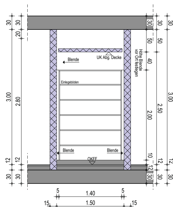
Wandansicht A
