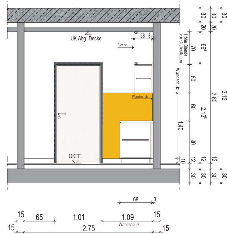
Wandansicht B
