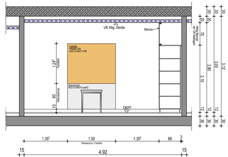
Wandansicht C
