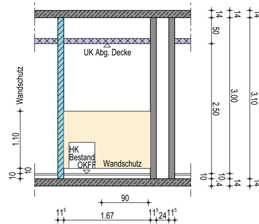
Wandansicht A
