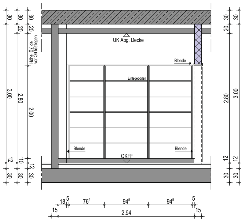
Wandansicht C
