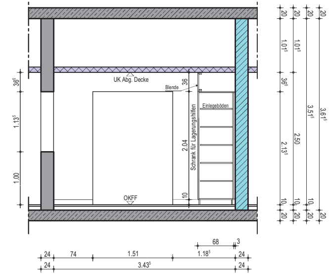
Wandansicht B
