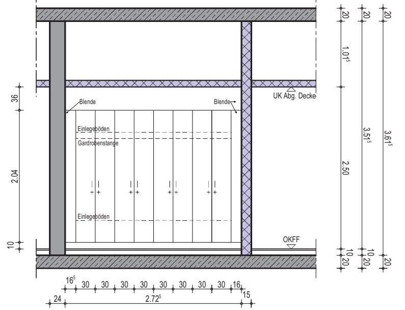
Wandansicht D
