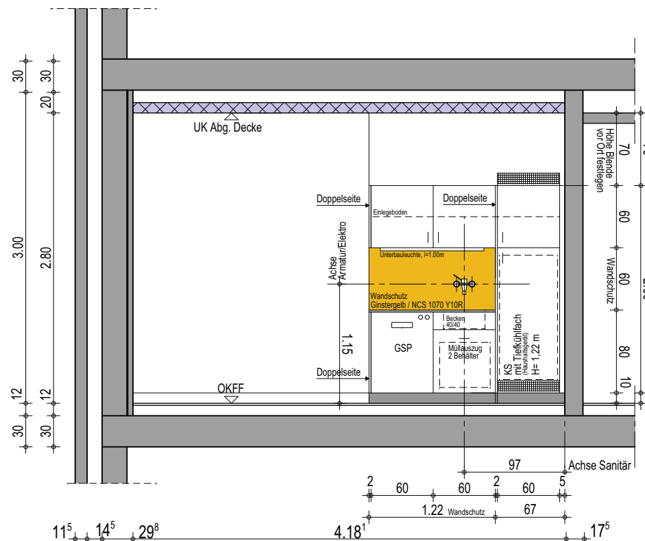
Wandansicht A
