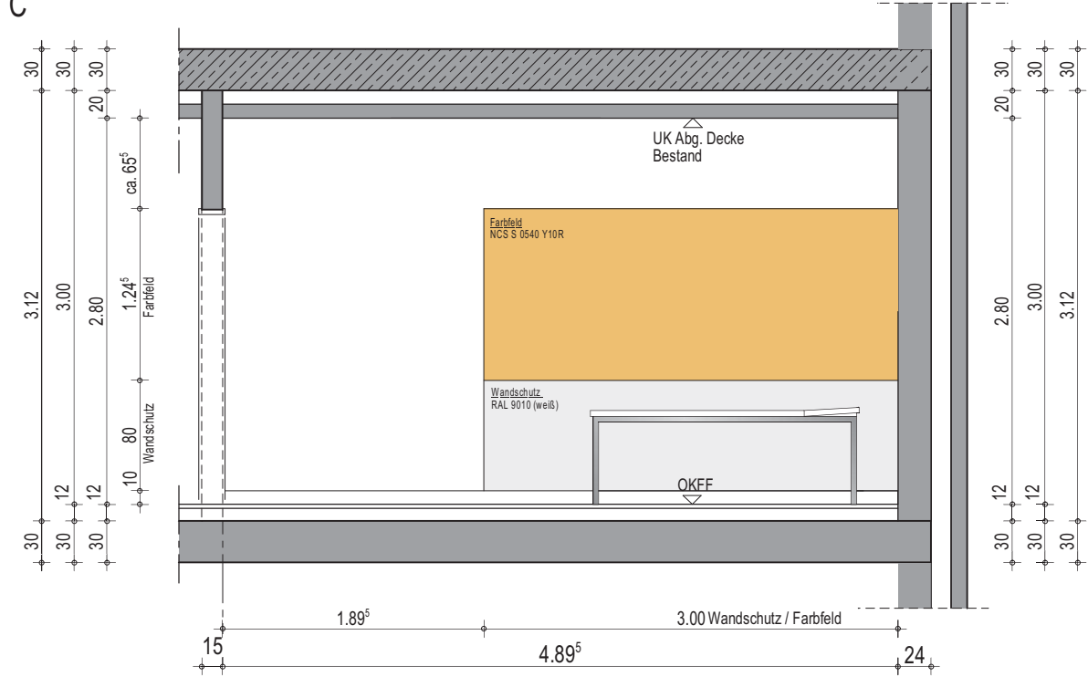
Wandansicht C
