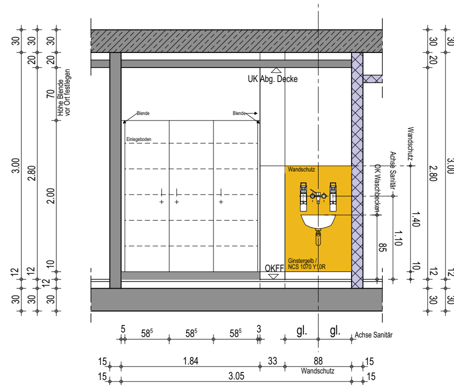
Wandansicht A
