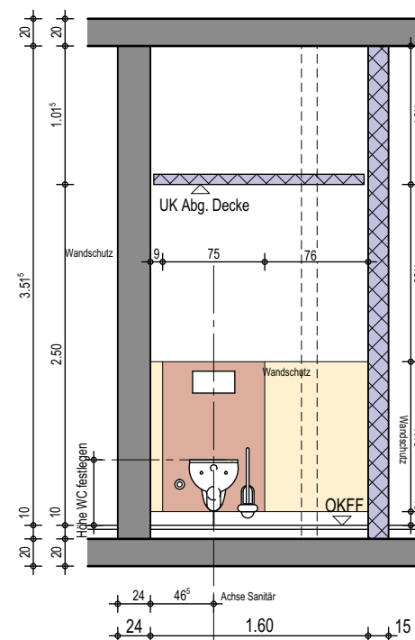
Wandansicht A
