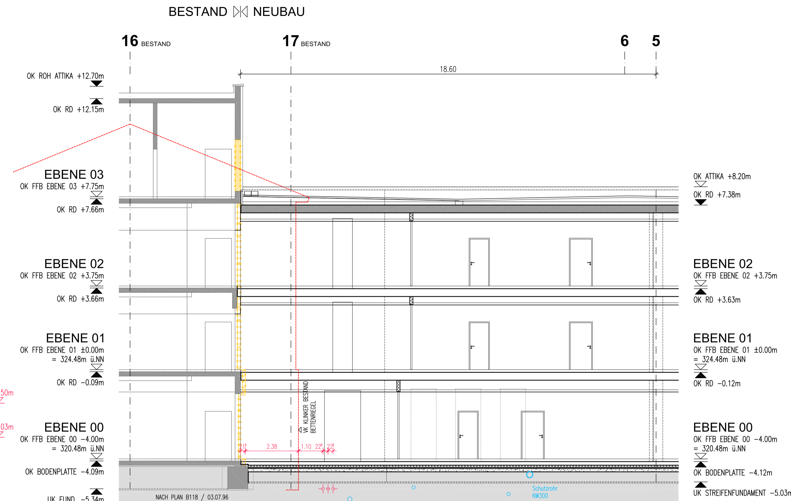
SCHNITT CC
