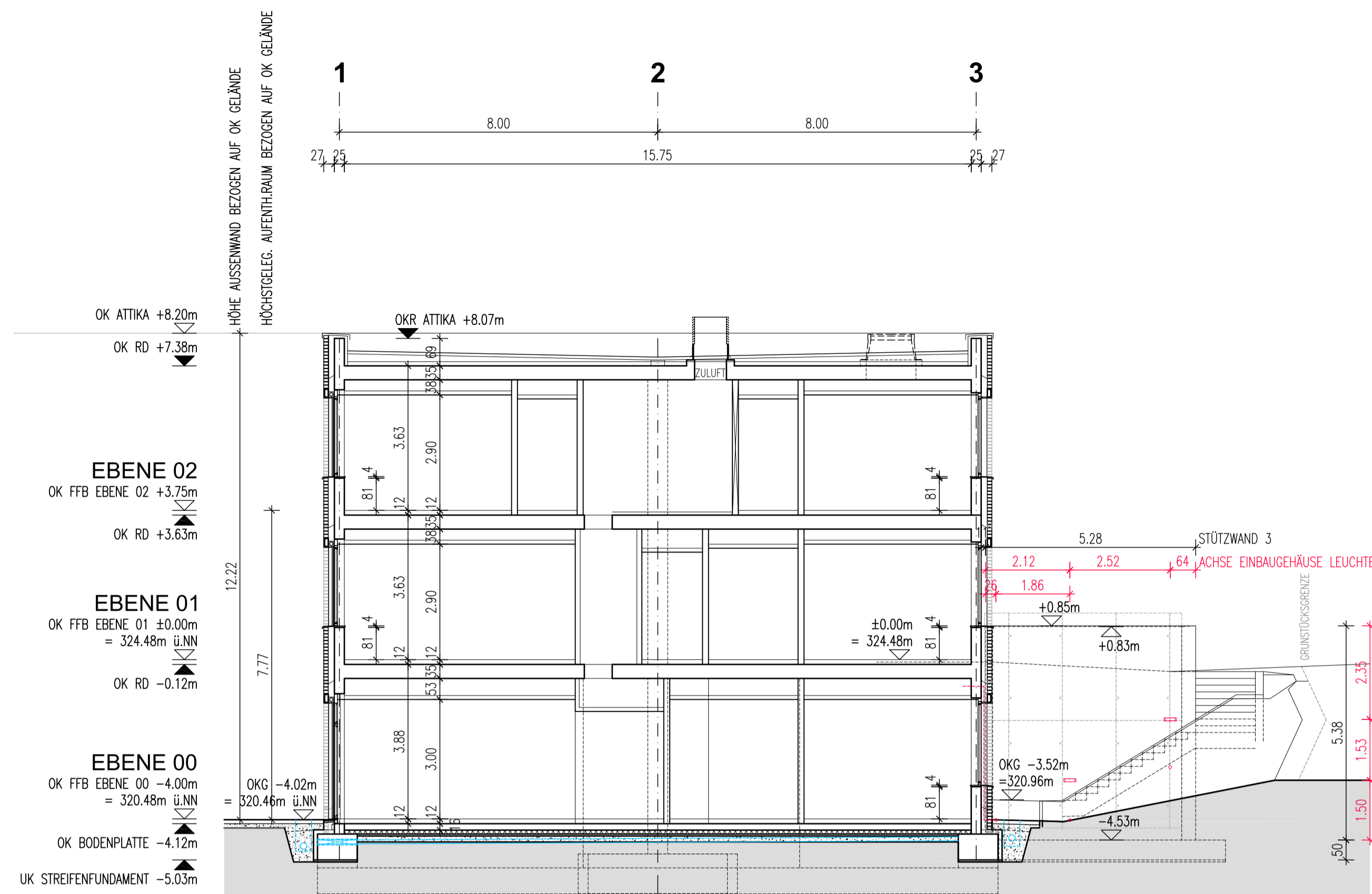
SCHNITT BB
