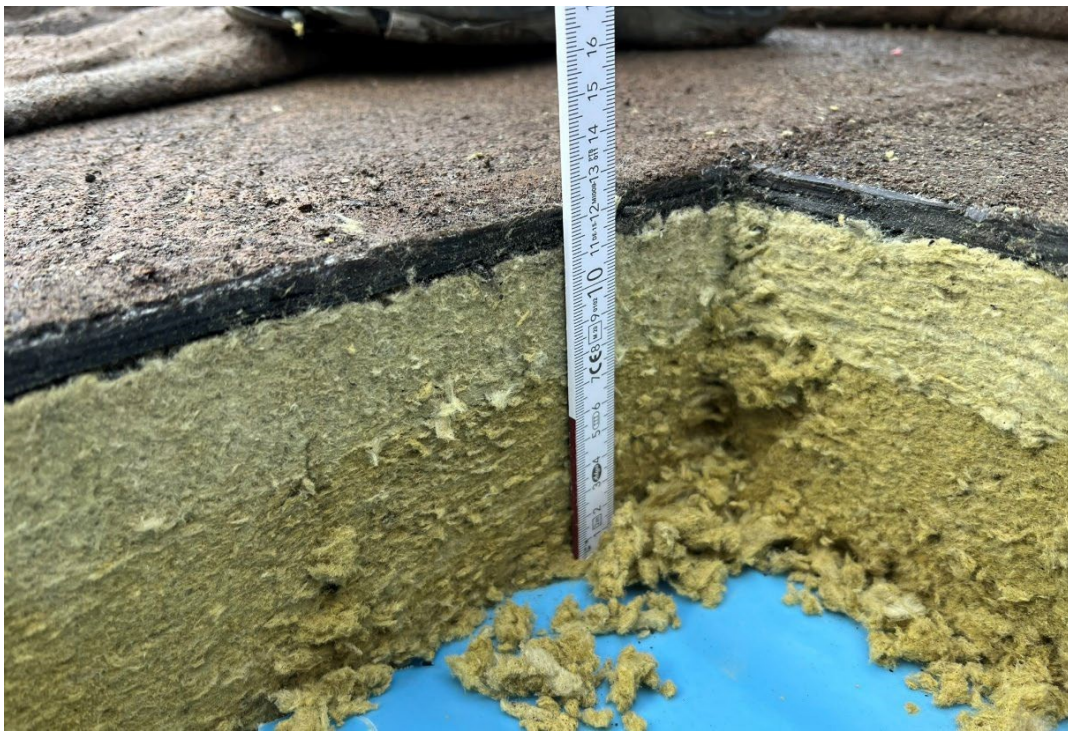
Abb. 19: Dachaufbau 6 – Höhe Dämmschicht
