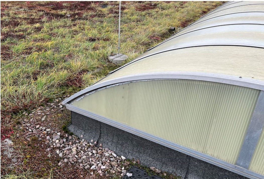
Abb. 5: Zustand Lichtbänder 2
