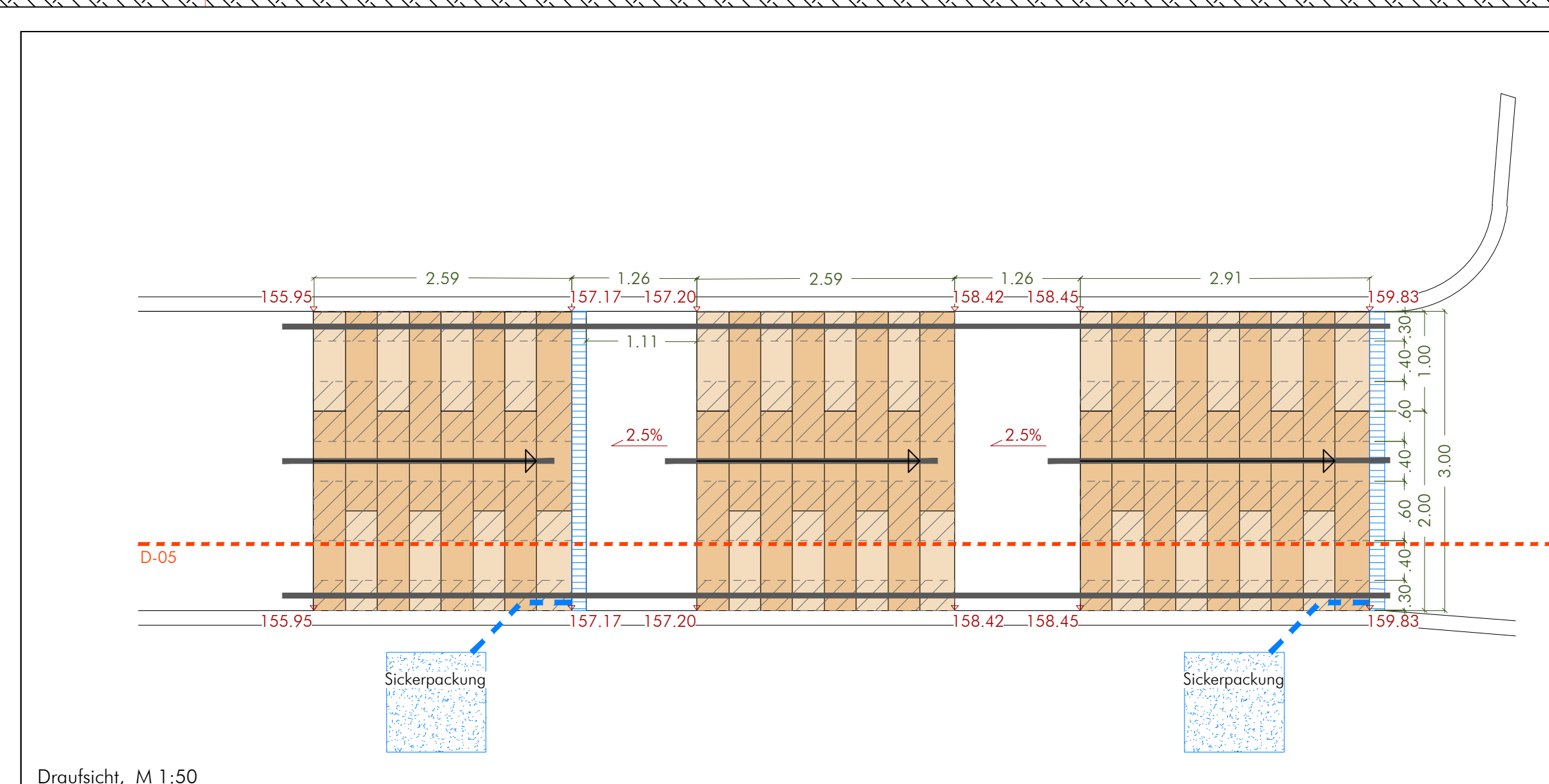
Draufsicht, M 1:50
