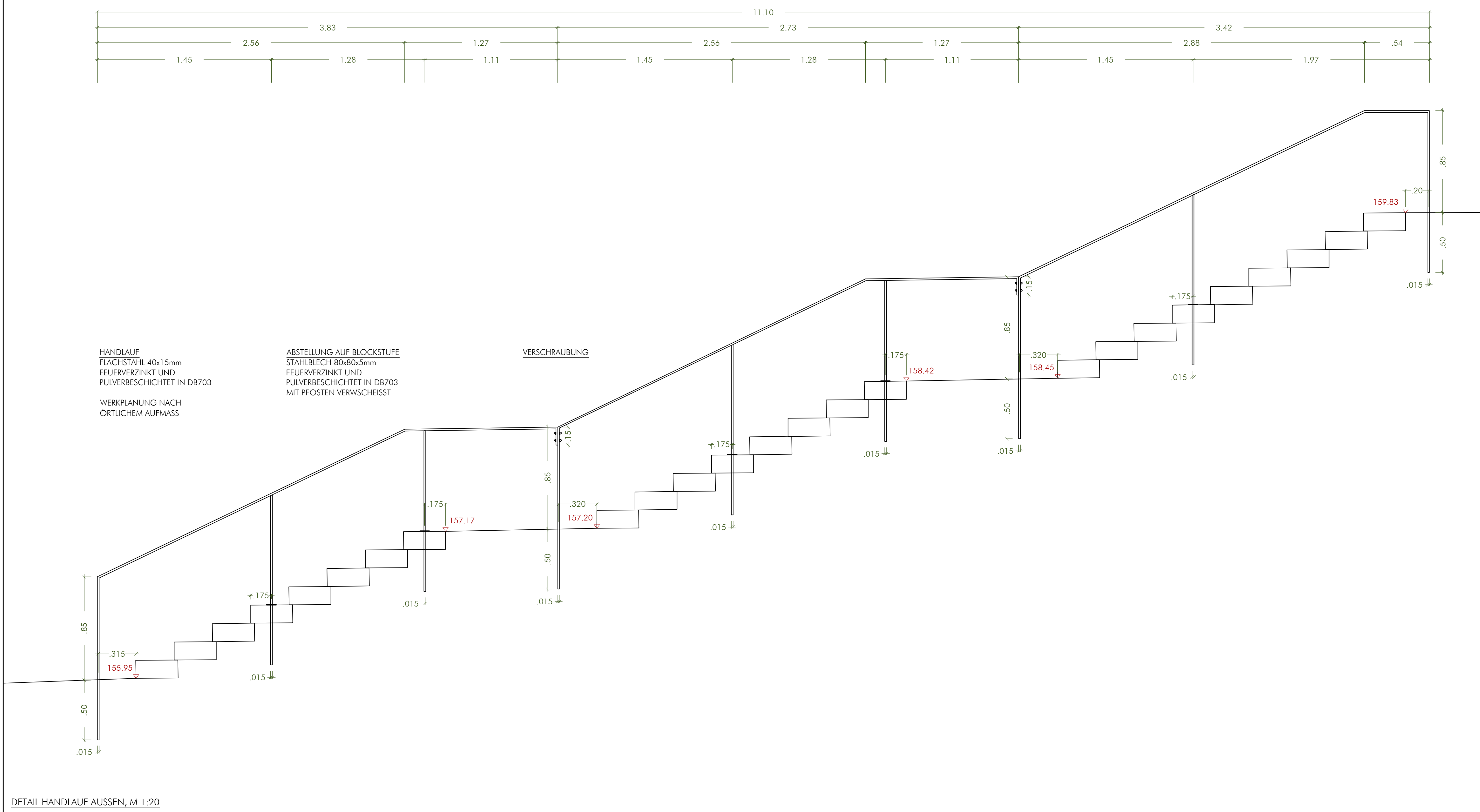
DETAIL HANDLAUF AUSSEN, M 1:20
