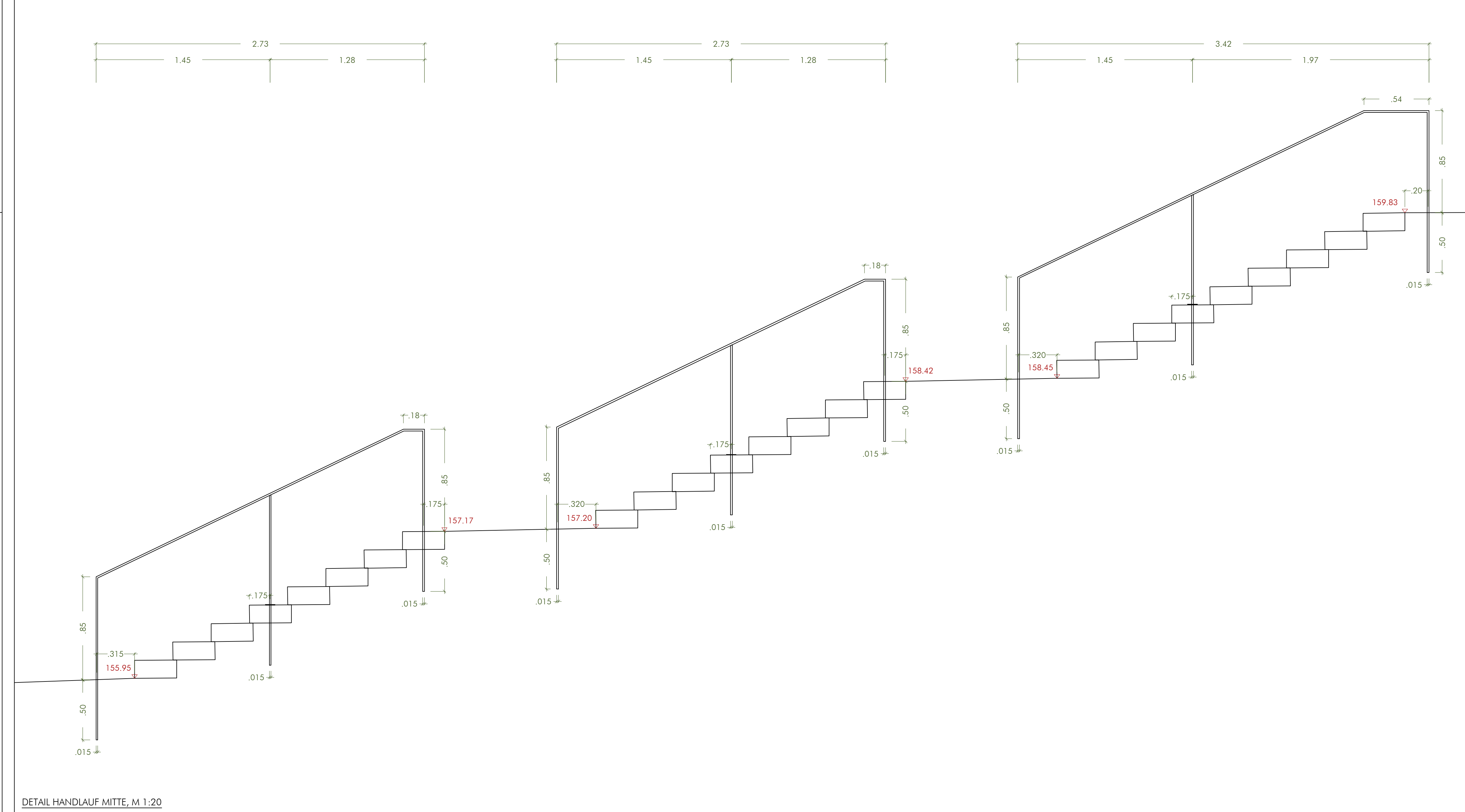
DETAIL HANDLAUF MITTE, M 1:20
