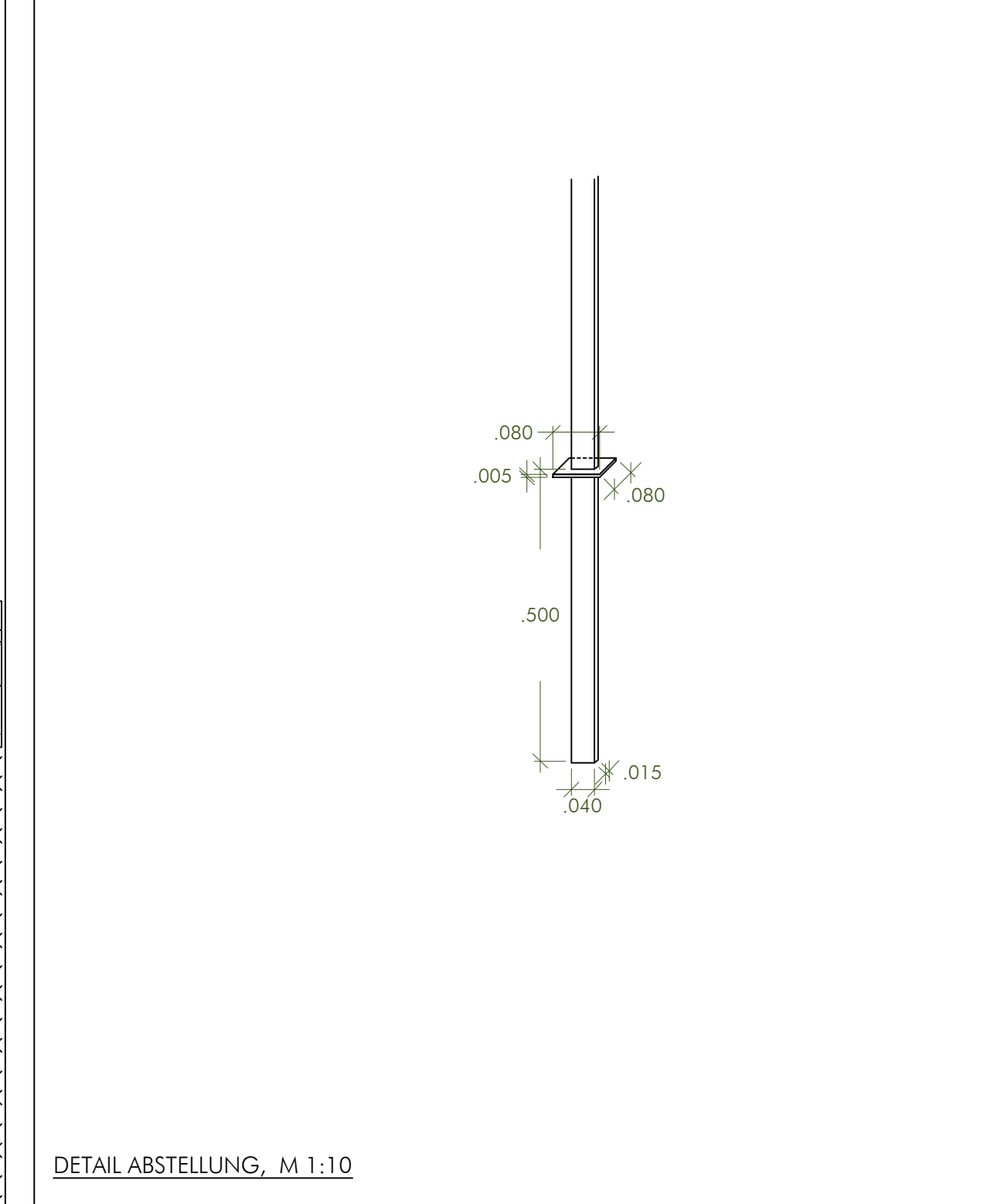
DETAIL ABSTELLUNG, M 1:10
