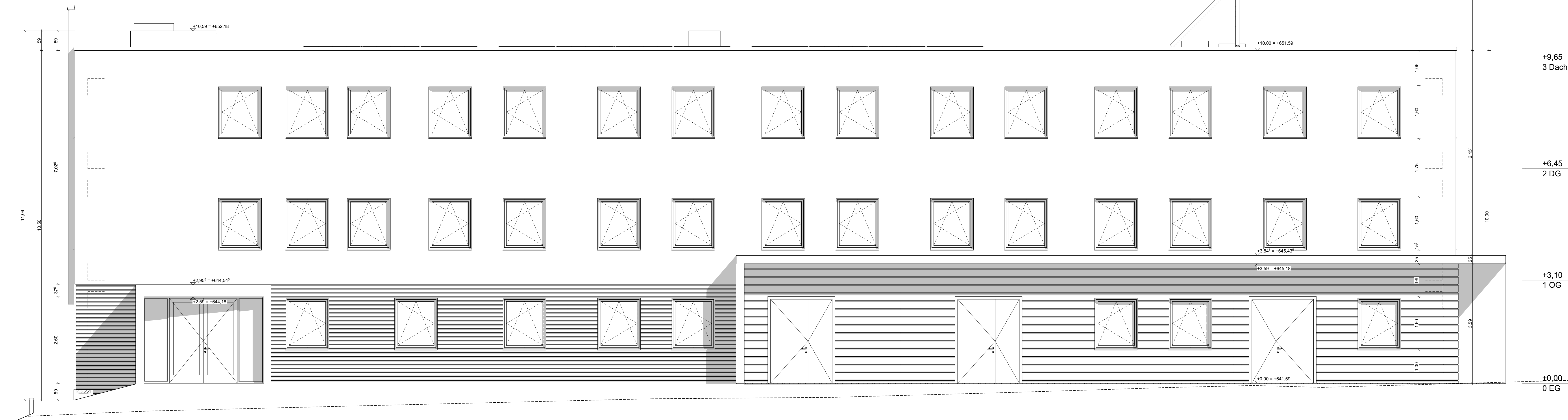
A-04 Ansicht West 1:50
