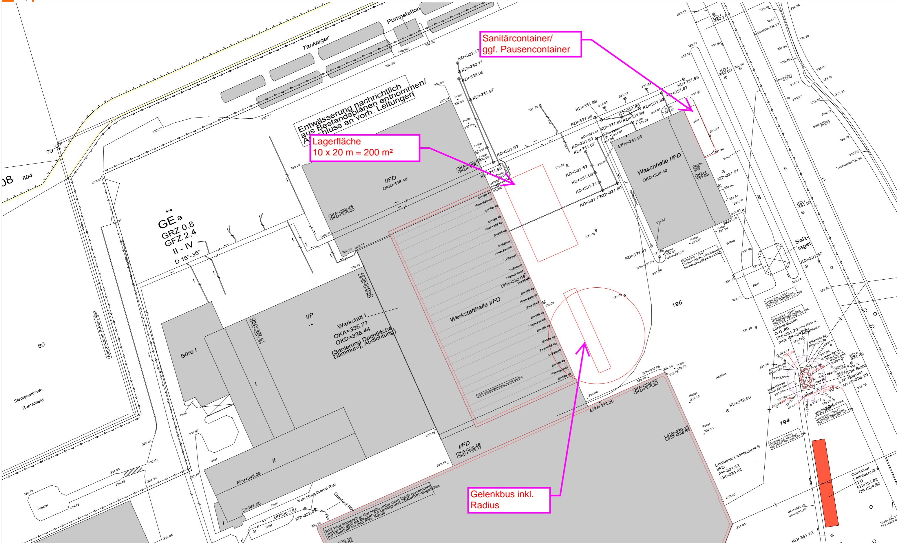
23013 Stadtwerke RS, Dacherrhöhung Werkstatthalle - Lageplan M 1 : 500 | Stand 15.03.2024
