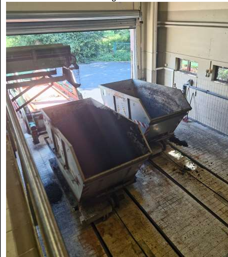
Abb. 2: Klärschlammverladung
