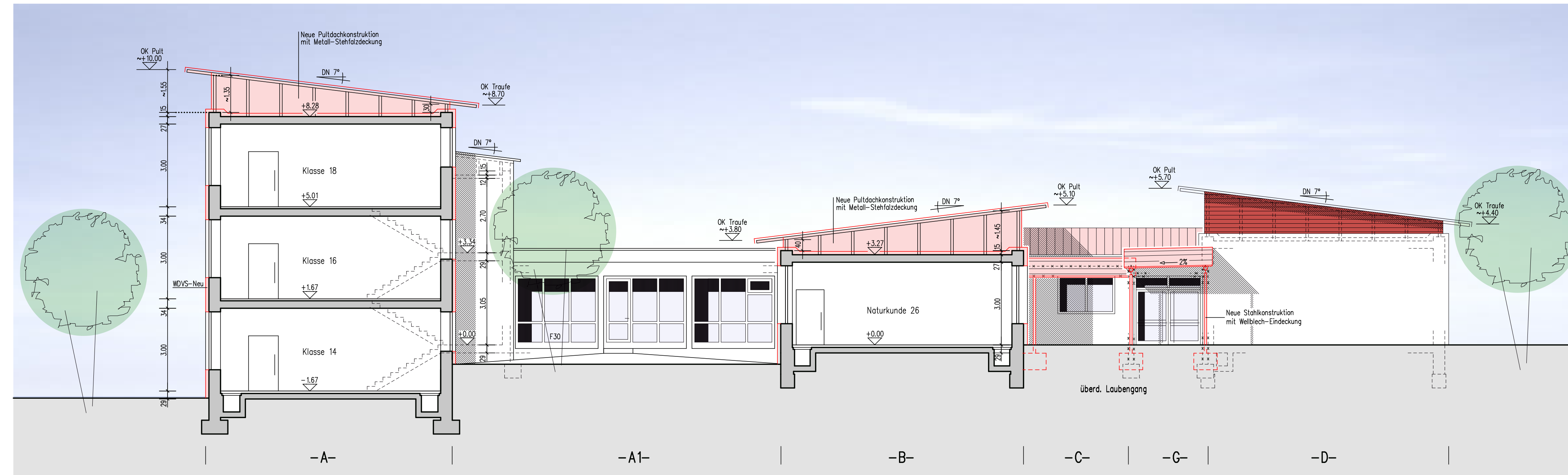
Schnitt A-A
