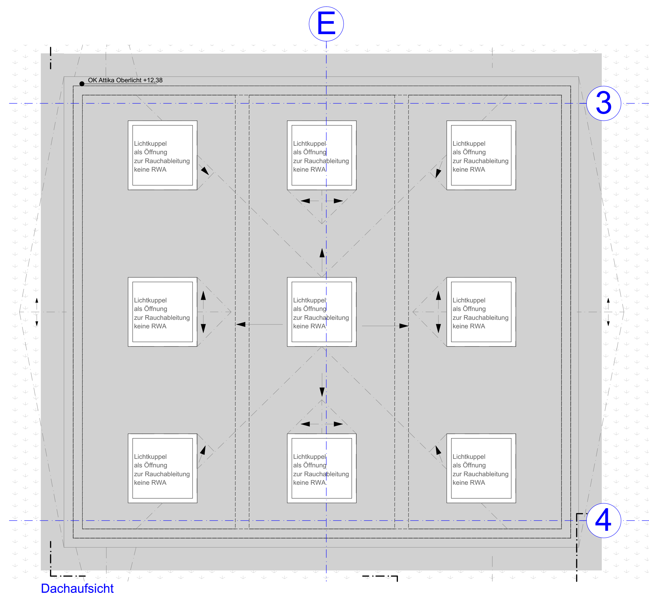
Dachaufsicht
