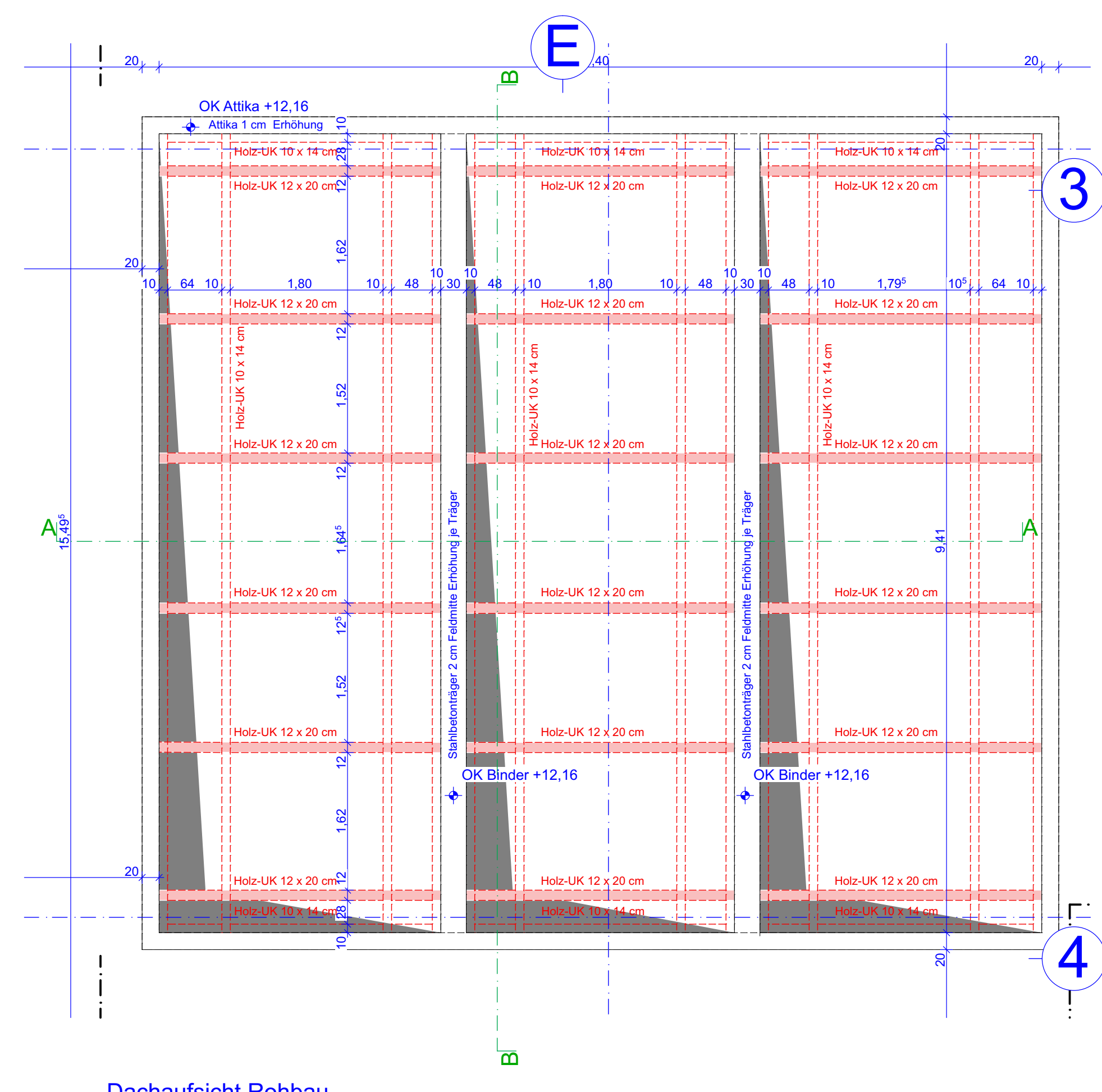
Dachaufsicht Rohbau
