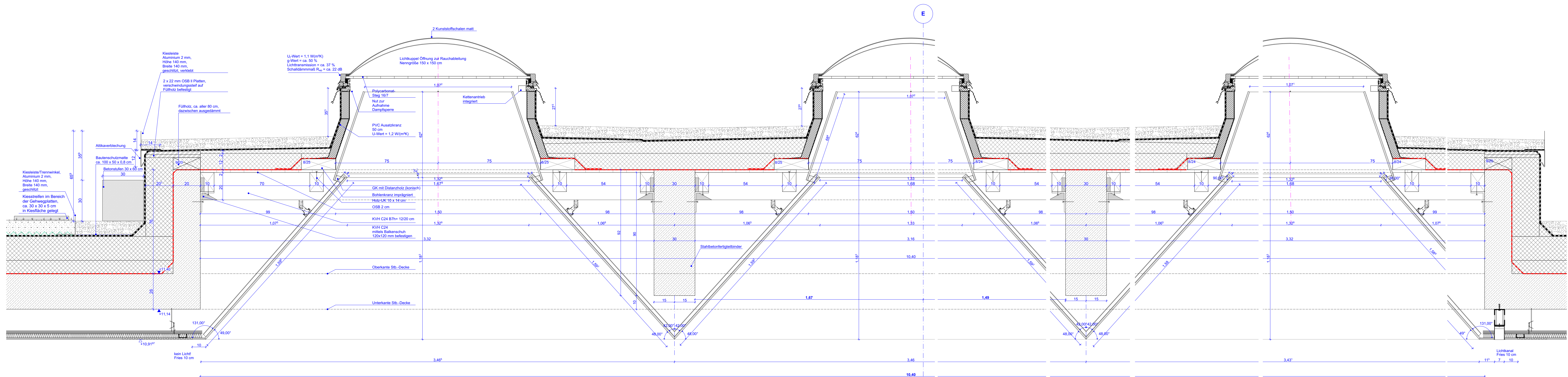
Schnitt B-B Längs
