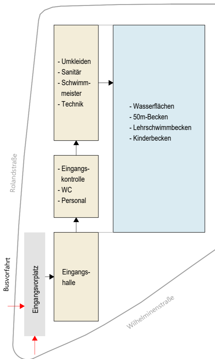
Erdgeschoss
