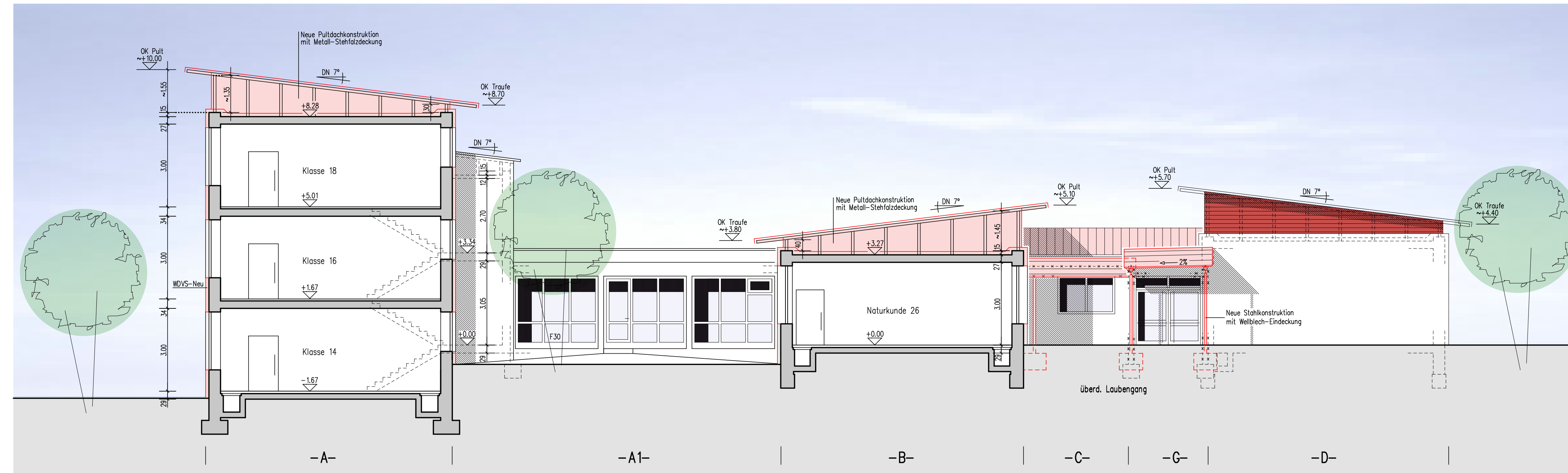
Schnitt A-A
