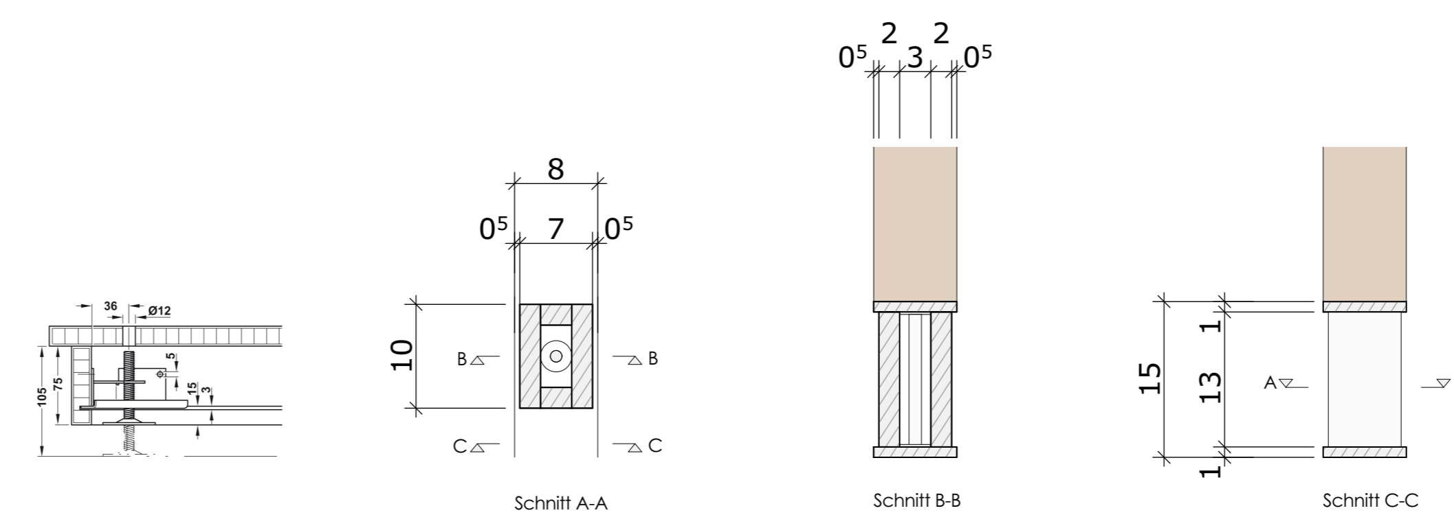
Sockeldetail zu Typ 2.2 M 1:5
