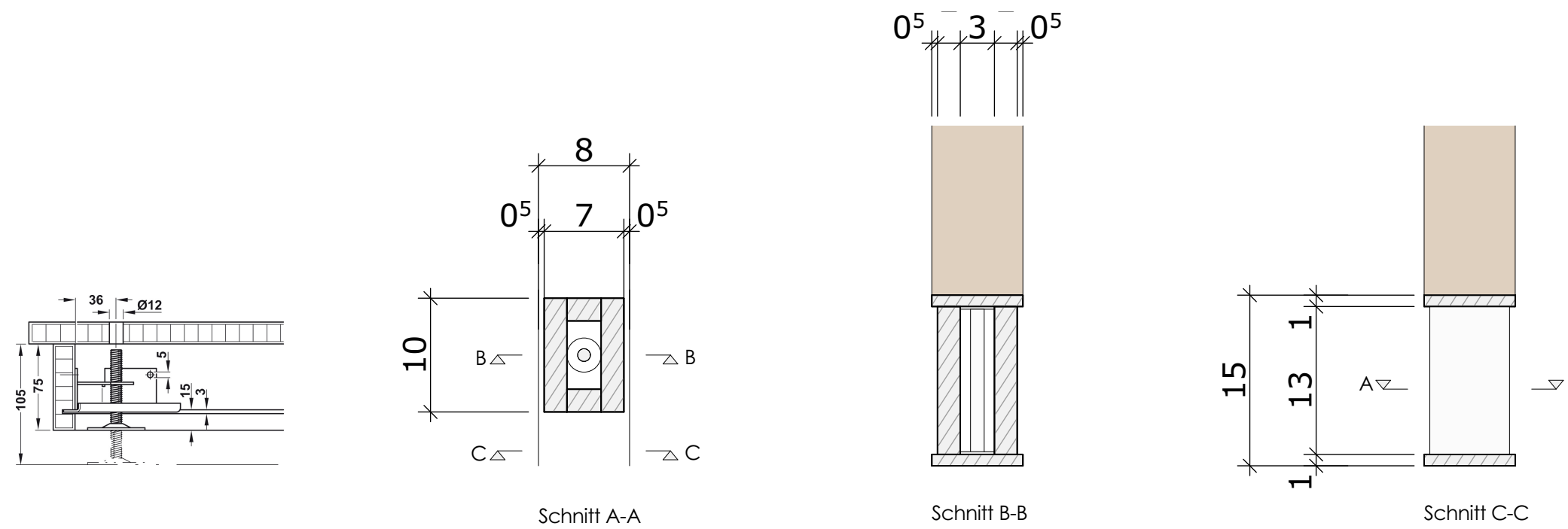
Sockeldetail zu Typ 2.2 M 1:5
